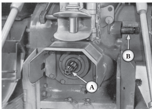
A — محور انتقال نیرو ۶ شپاره — محور انتقال نیرو، یدکی ۲۱ شپاره
